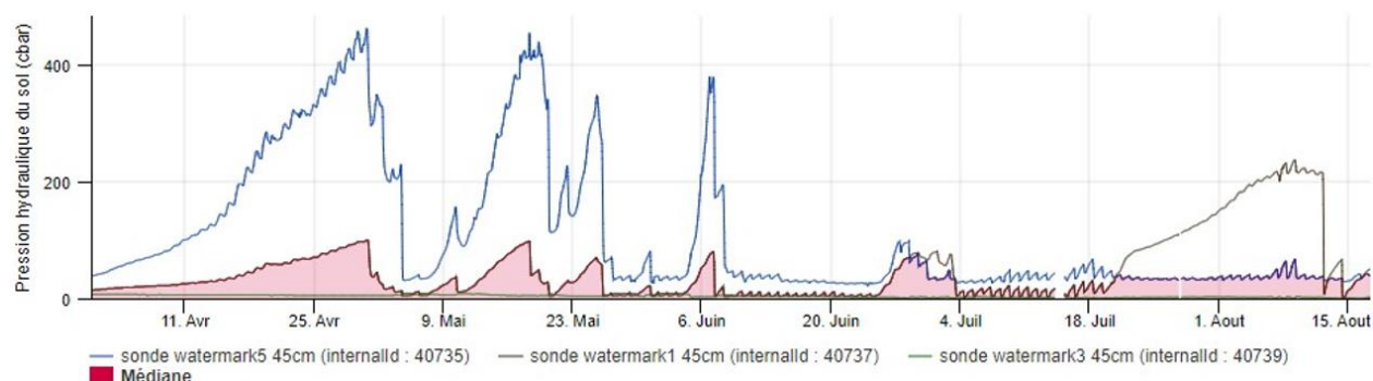
Figure 45 : Evolution de la pression hydraulique de M1 à 45cm de profondeur du 1 er Mai au 25 août 2022
