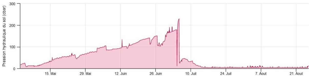
Figure 68 : Evolution de la pression hydraulique de M1 à 75cm de profondeur du 1 er Mai au 25 août
