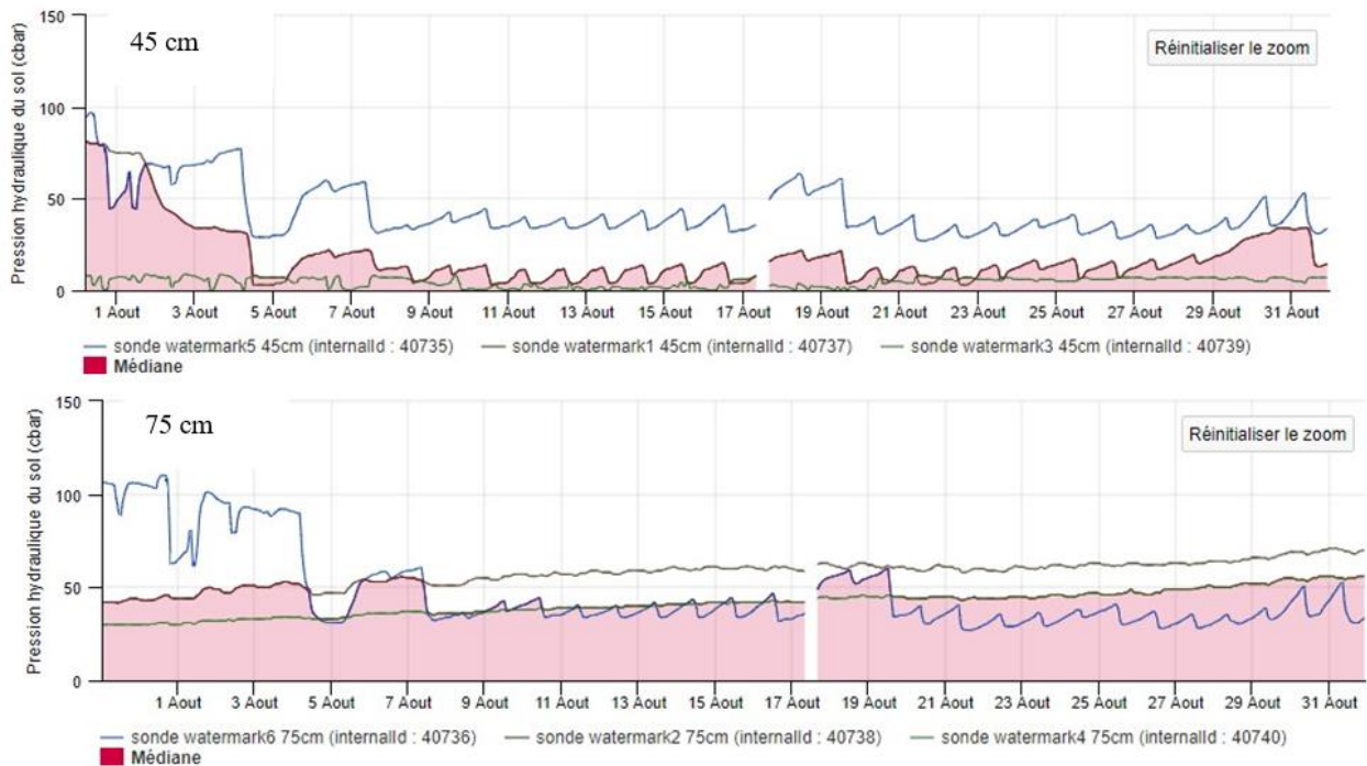
Figure 30 : Courbe de pression hydraulique mesurées par les sondes Watermarks à 45 cm et 75 cm pour la modalité M1 en août 2021
