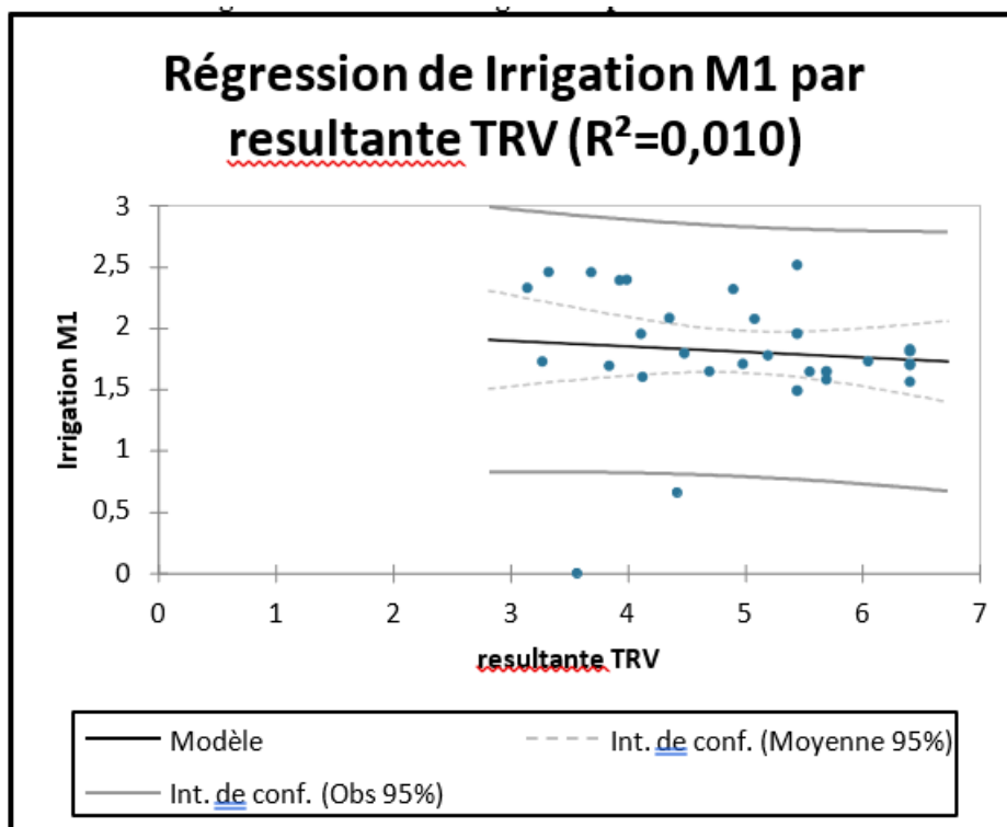
Figure 52 : courbe de régression pour l'indice TRV
