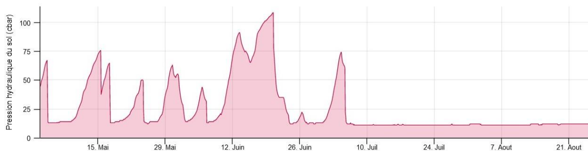
Figure 71 : Evolution de la pression hydraulique de M3 à 45cm de profondeur du 1er Mai au 25 août
