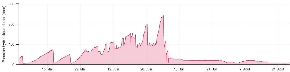
Figure 67 : Evolution de la pression hydraulique de M1 à 45cm de profondeur du 1 er Mai au 25 août
